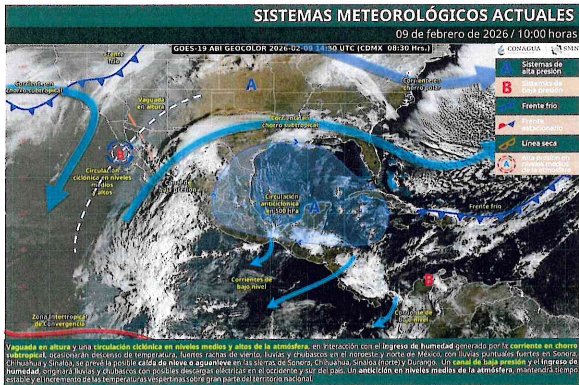
Fig. 1. Sistemas meteorológicos actuales.
