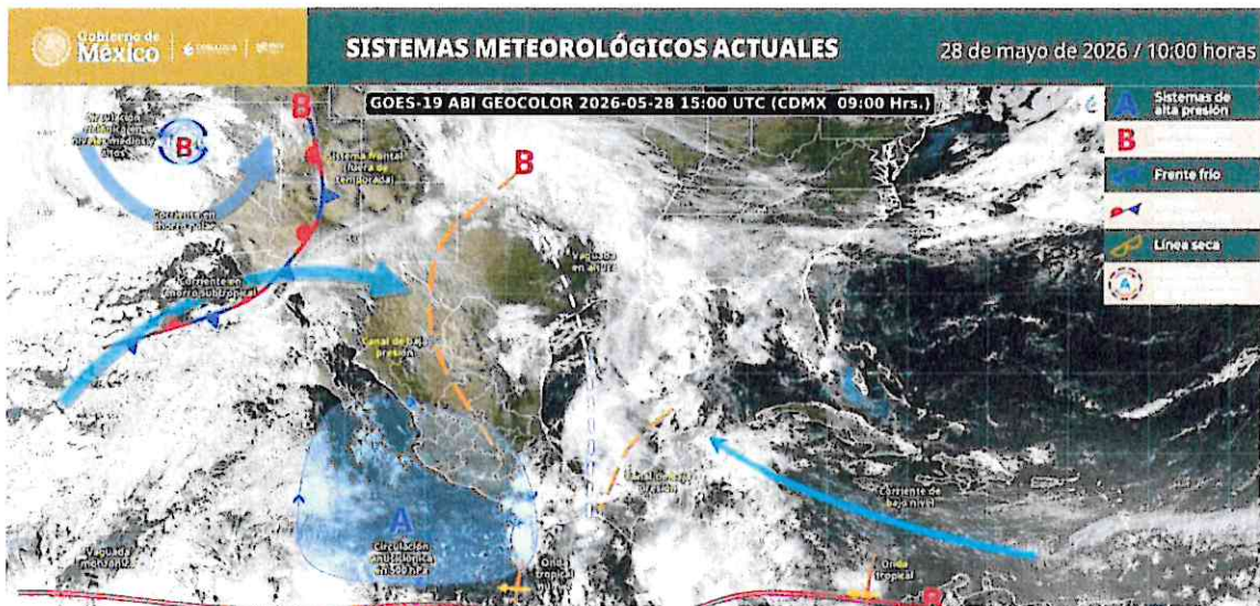
Fig. 1. Sistemas meteorológicos actuales.
